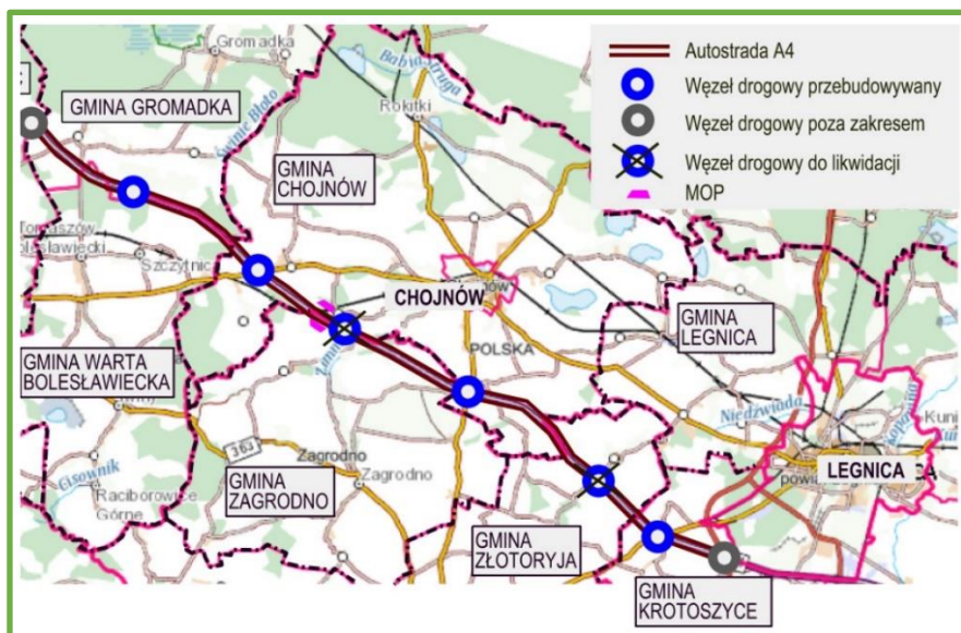
Rysunek 6. Projekt przebudowy/likwidacji węzłów autostradowych w ciągu autostrady A4 (odcinek Krzyżowa - Legnica Południe), materiały GDDKiA ze spotkania informacyjnego dla Gminy Chojnów i Gminy Zagrodno, grudzień 2022.r.
